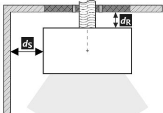
Подключение заднего дымохода
